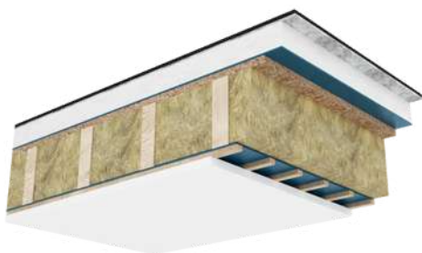
DECKE
